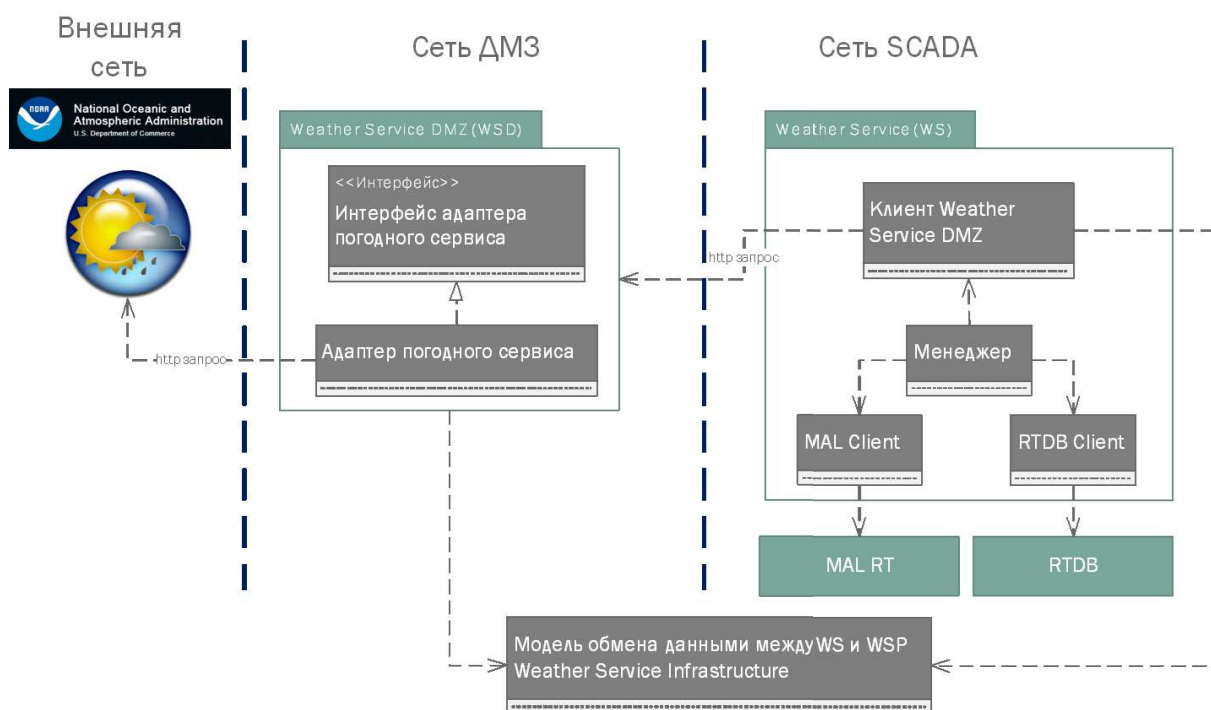
Архитектура службы метеоданных
